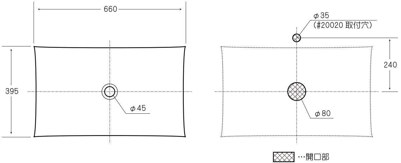
カウンター開口寸法の目安 （#20020、HL-4534 使用の場合）
